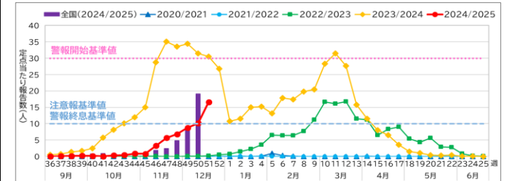
図1 定点当たり報告数 (全国及び山形県過去4シーズンとの比較)
